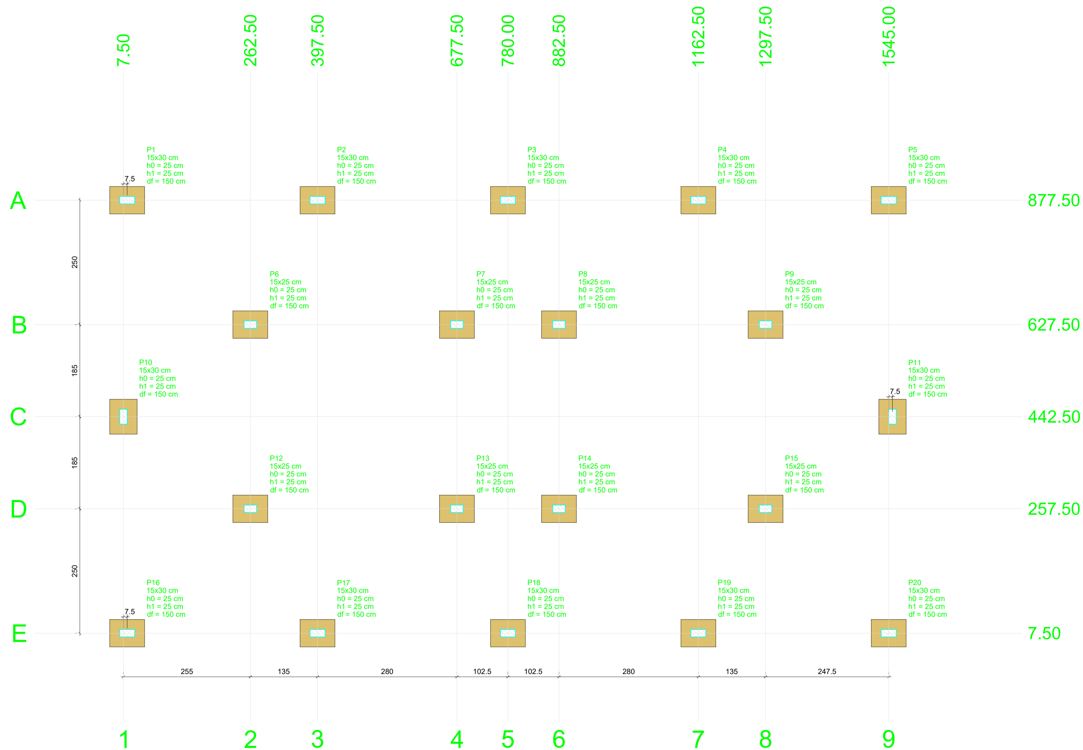
Planta de localização escala 1:50
