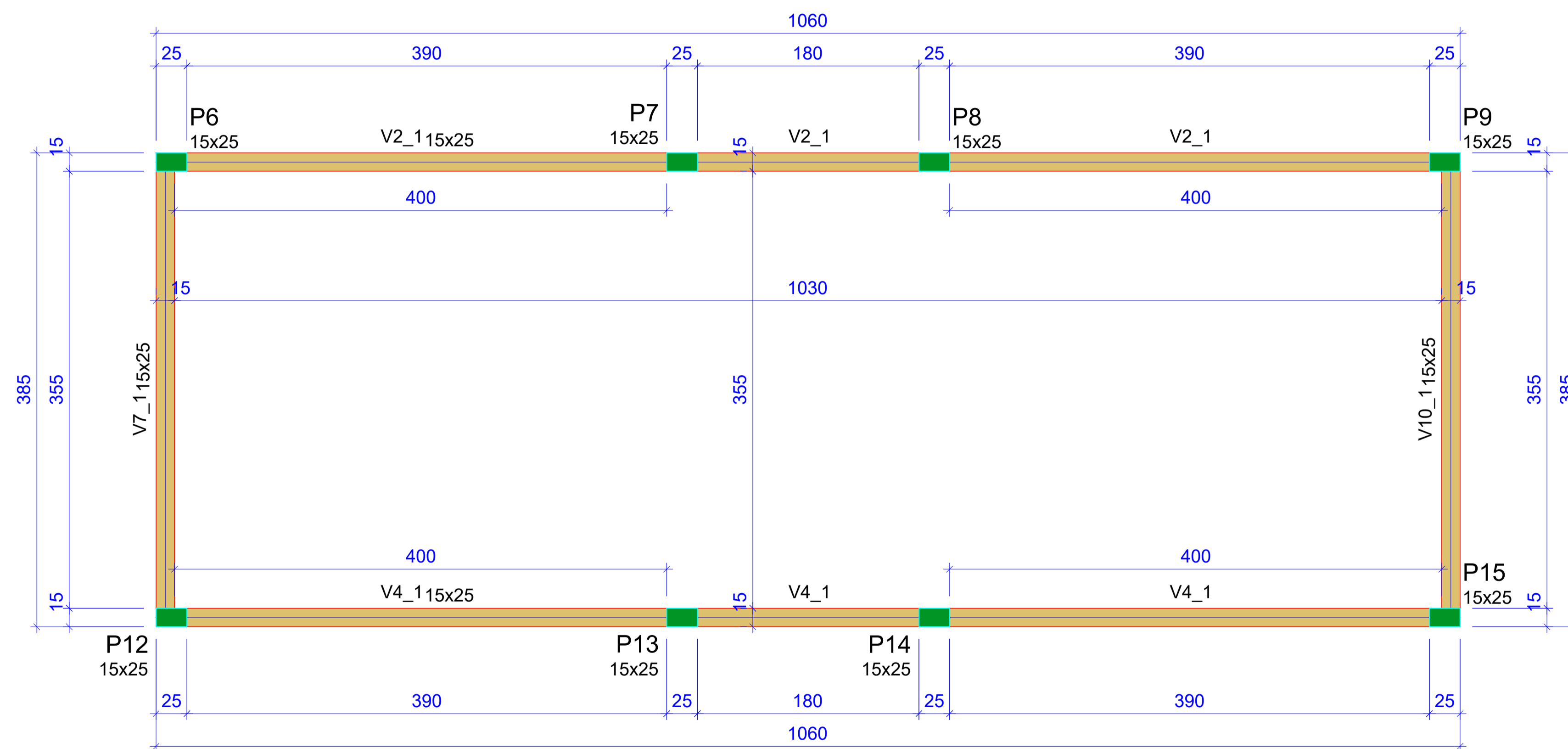
Forma do pavimento Cintamento Final escala 1:50
